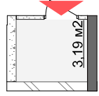
План приміщення тип 3
