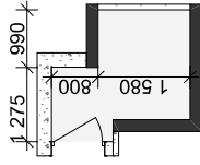
План приміщення з основними розмірами
